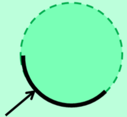
Arc
